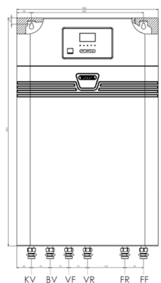
Tilslutningsskitse, højrevendt
